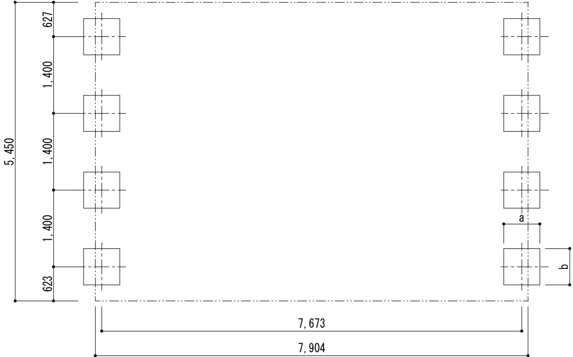
■ 基礎配置図
